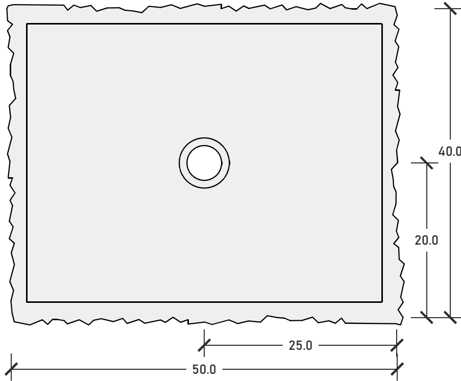
Pianta | Top
