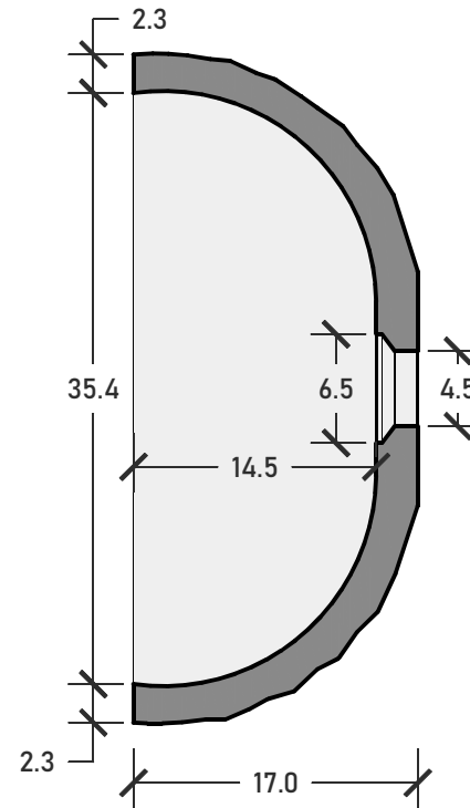
Sez. | Section
