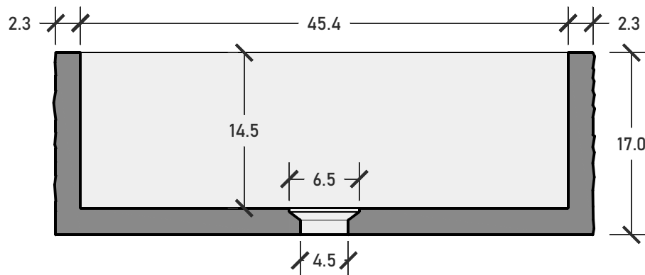
Sez. | Section
