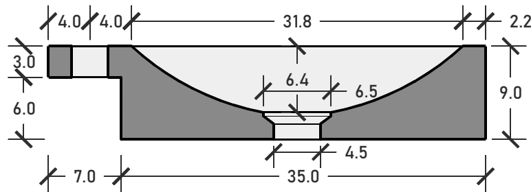
Sez. | Section
