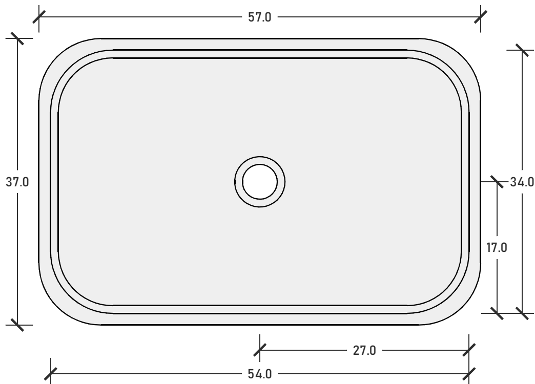
Pianta | Top
