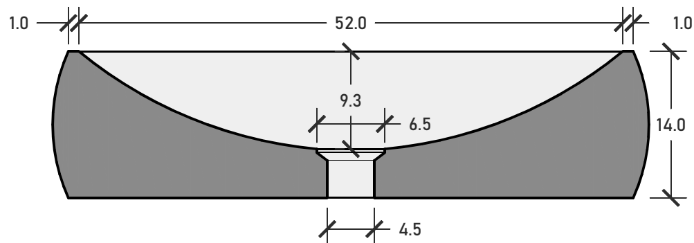
Sez. | Section
