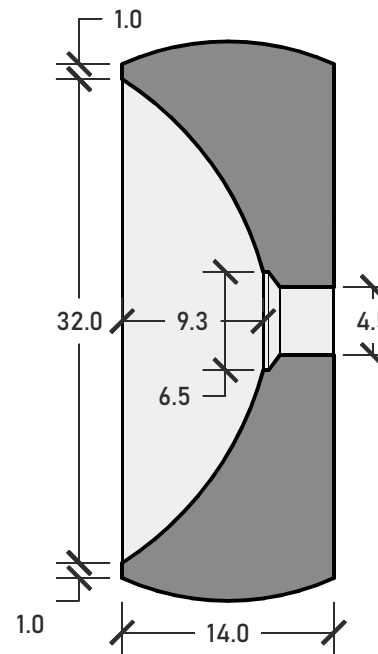
Sez. | Section
