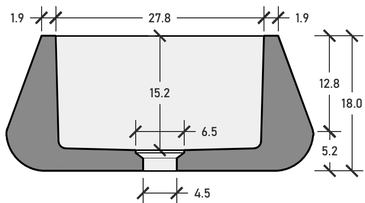
Sez. | Section
