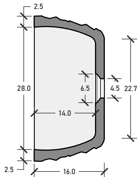
Sez. | Section
