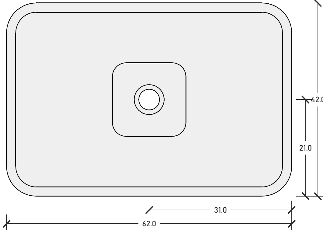
Pianta | Top
