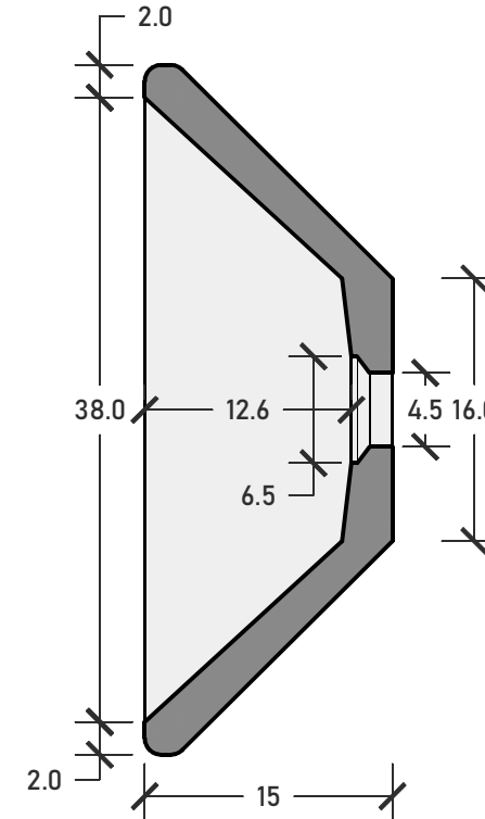
Sez. | Section
