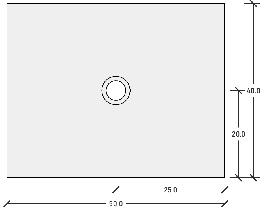
Pianta | Top
