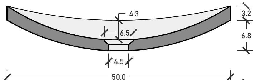
Sez. | Section
